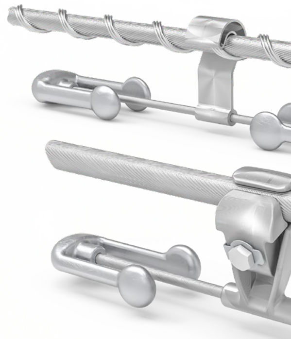
Stockbridge-Dämpfer mit Schraubbefestigung
